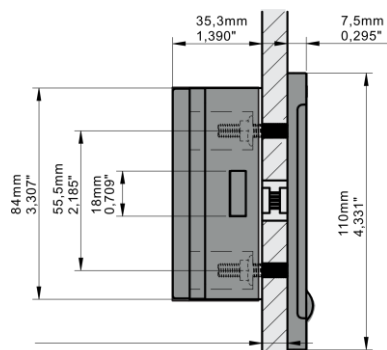
Vista perfil
