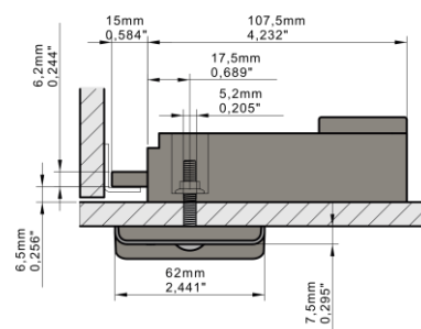
Vista alzado
