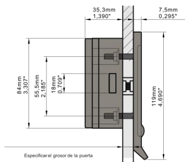
Vista perfil
