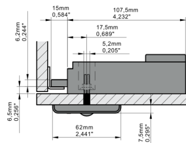
Vista alzado
