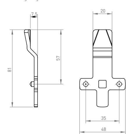
Fixing hole Einbaulochung
